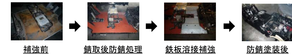
フレーム補修 溶接補強
